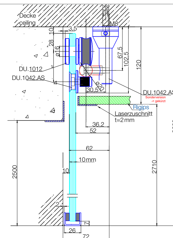
Technische Zeichnung der Laufschiene Technical drawing of the rail
